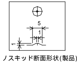
ノスキッド断面形状(製品)
