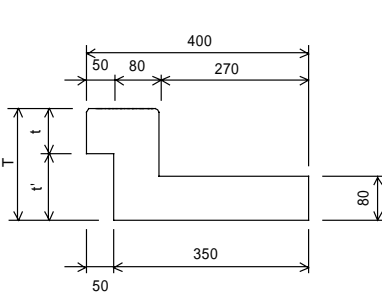
ノスキッド断面形状(製品)
